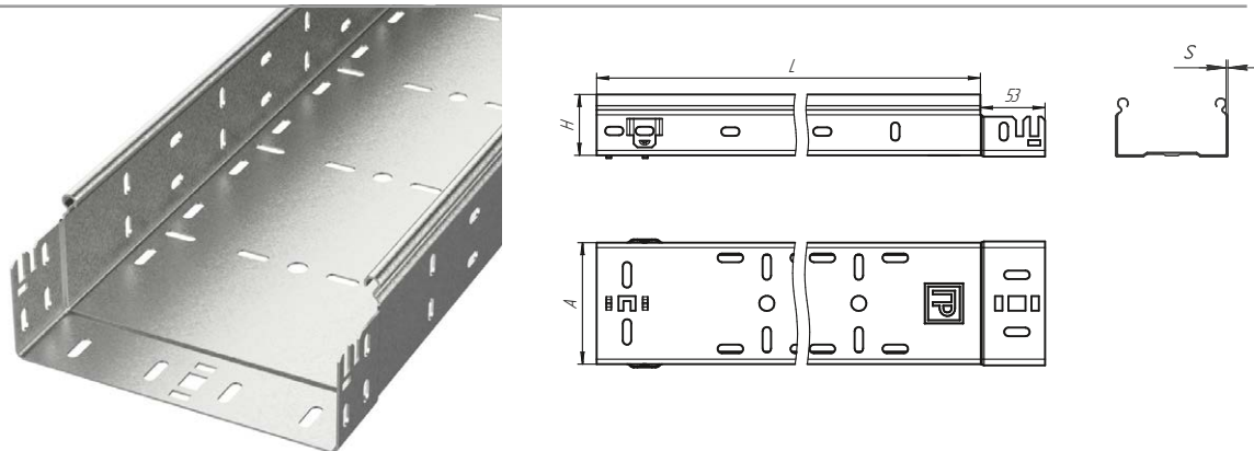
Лоток перфорированный Профи (1,0 мм)
