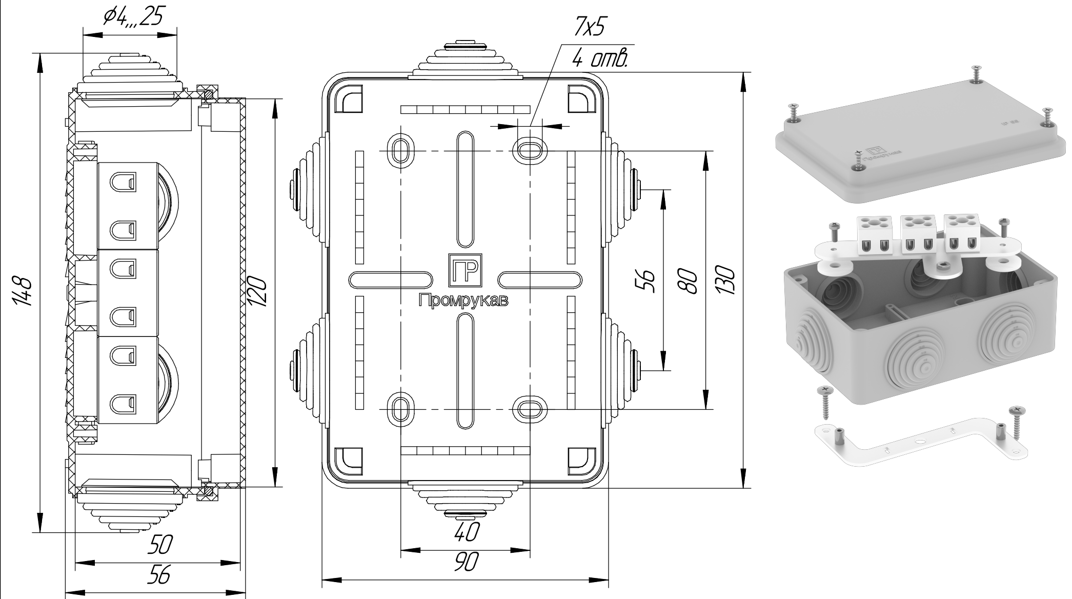
Коробка огнестойкая для о/п 40-0340-FR 120x80x50
